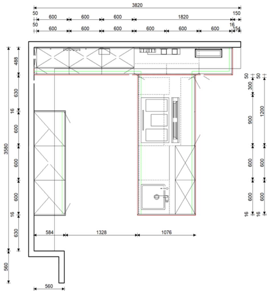
Cuisine d'exposition WT-38
