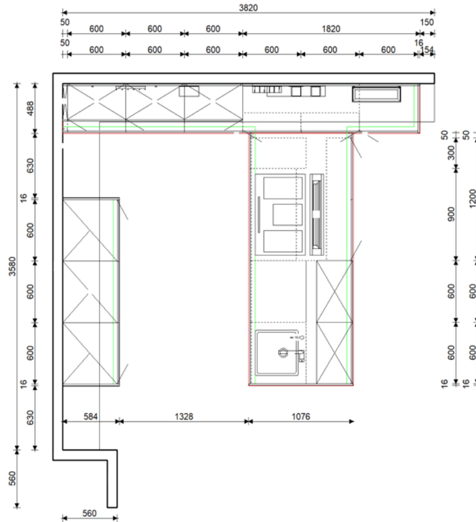
Musterküche WT-38
