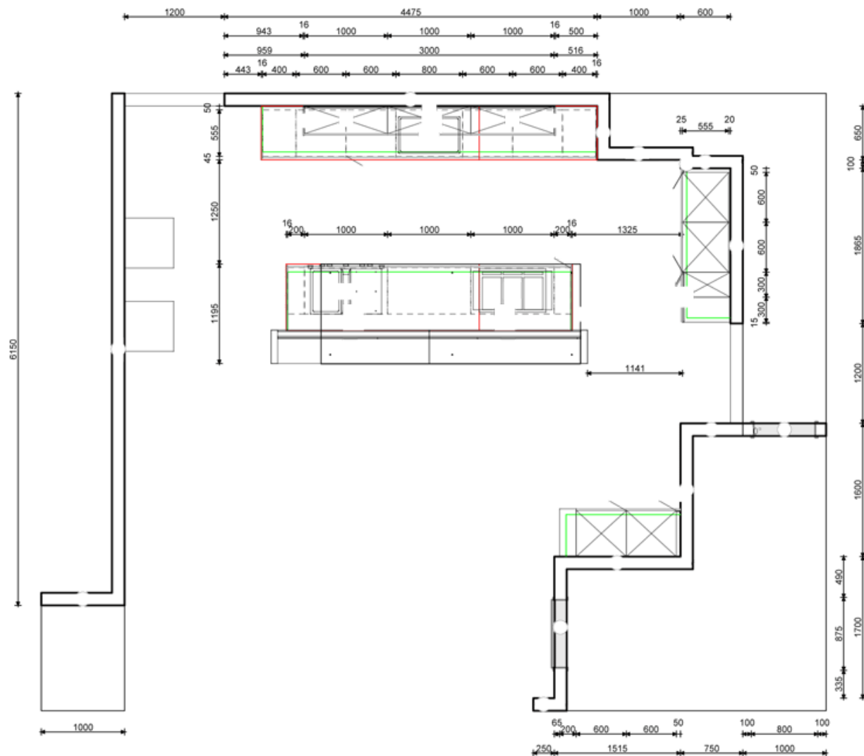
Cuisine d'exposition WT-24
