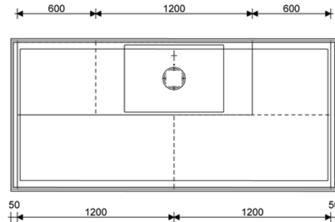
Musterküche WT-23
