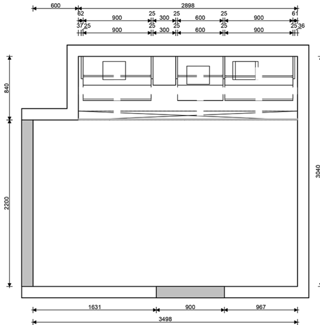
Musterküche WT-15B
