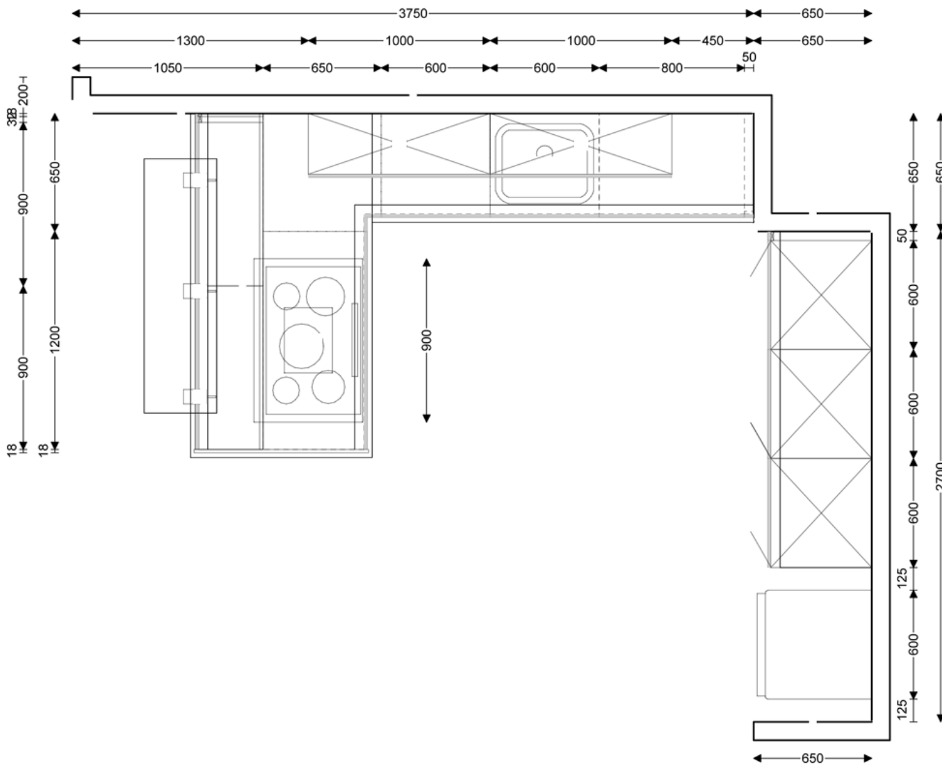
Cuisine d'exposition WT-12
