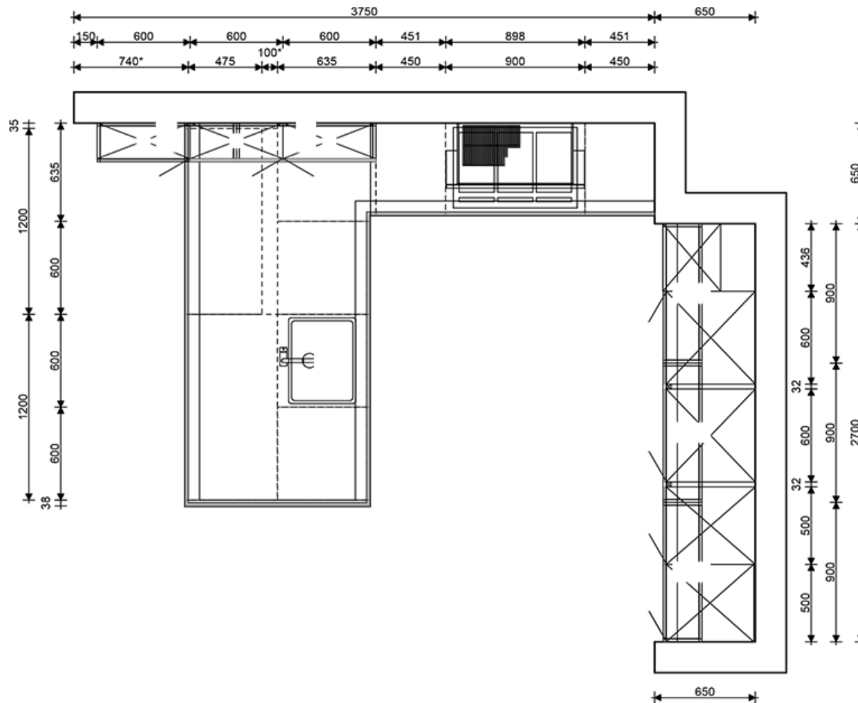
Musterküche WT-12
