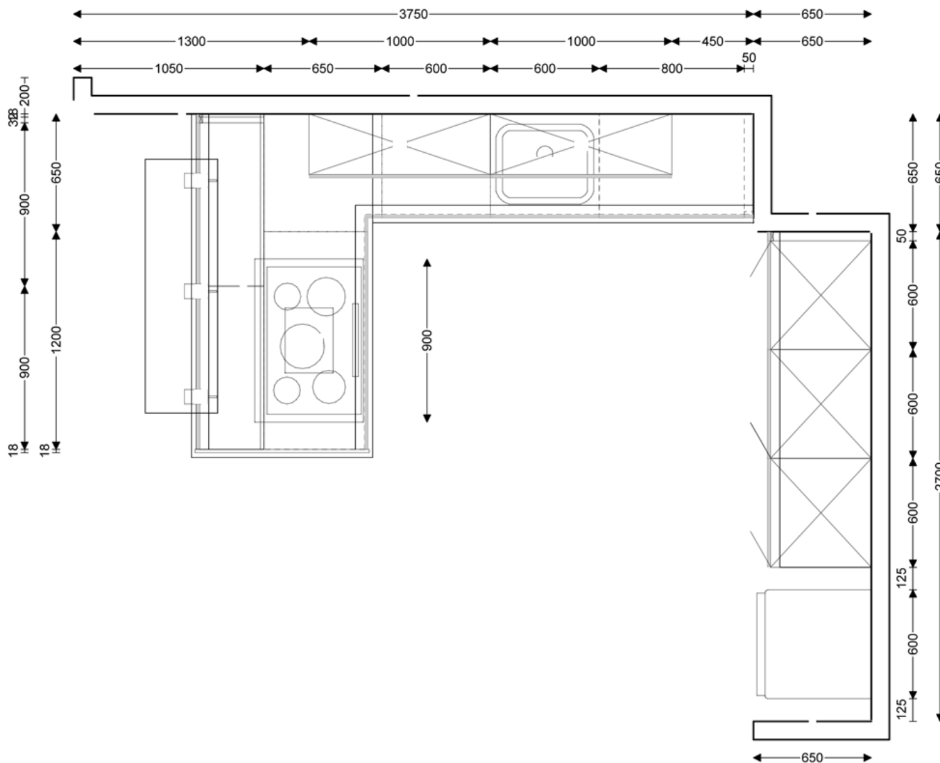
Musterküche WT-12
