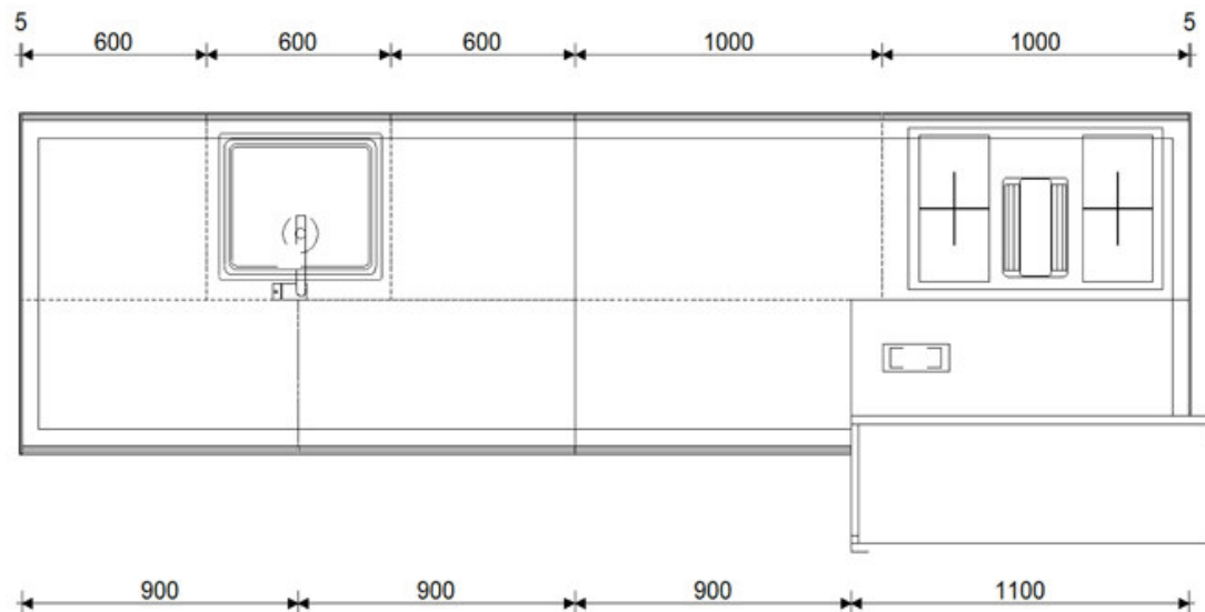
Musterküche RA-30
