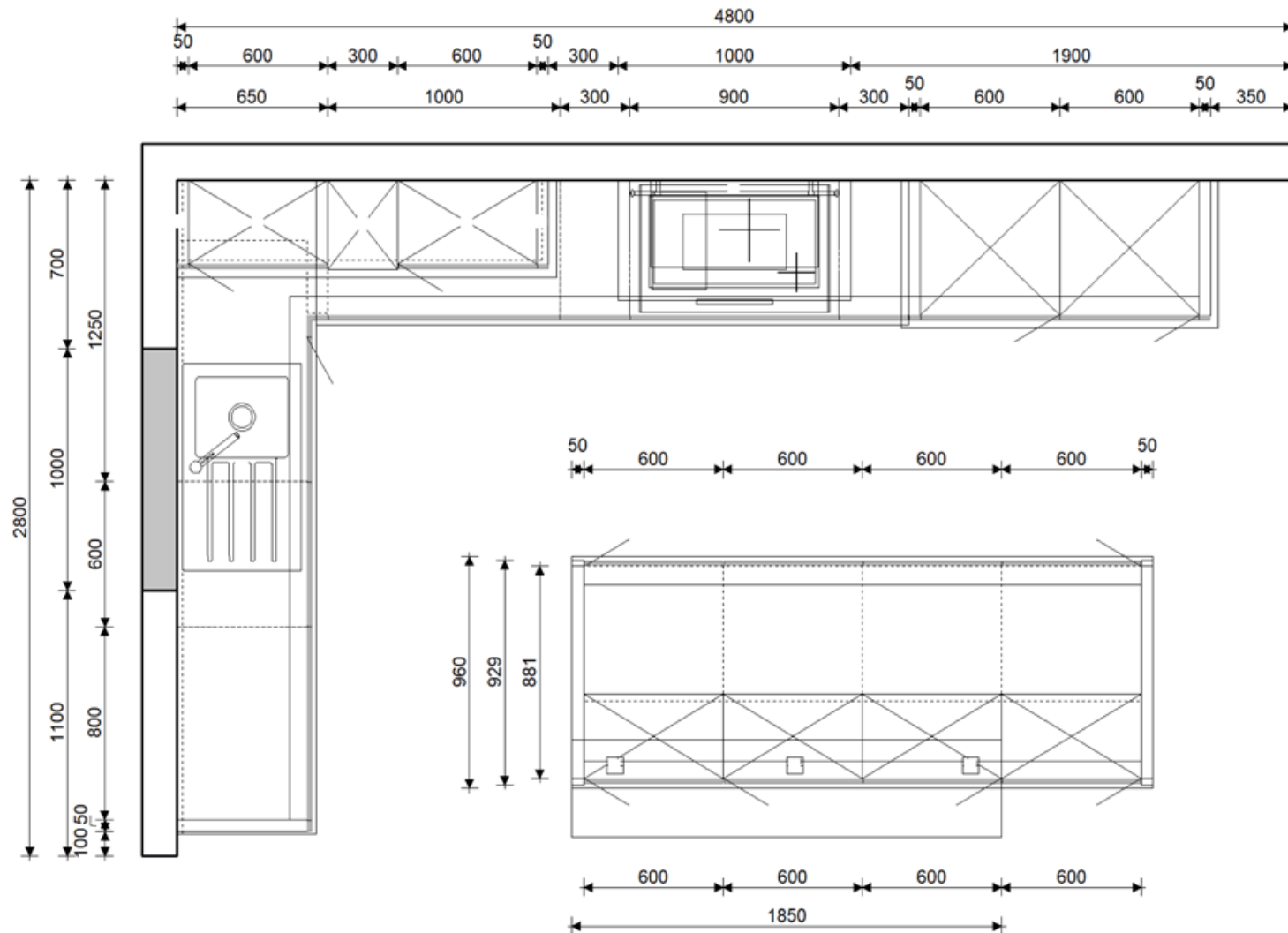
Musterküche RA-16
