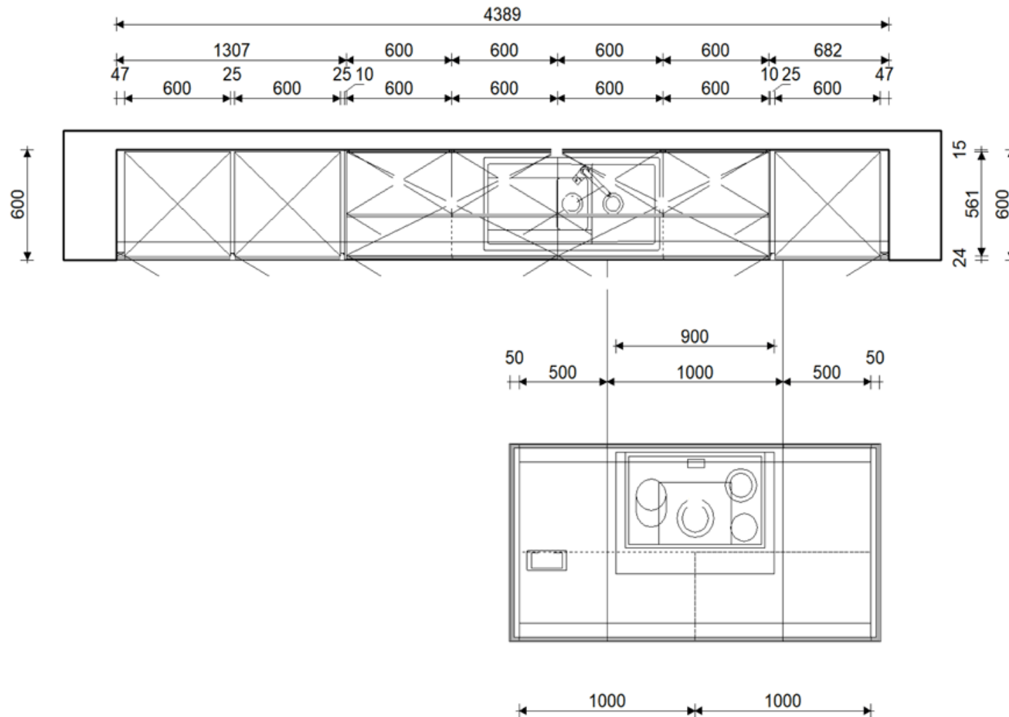
Cuisine d'exposition RA-15
