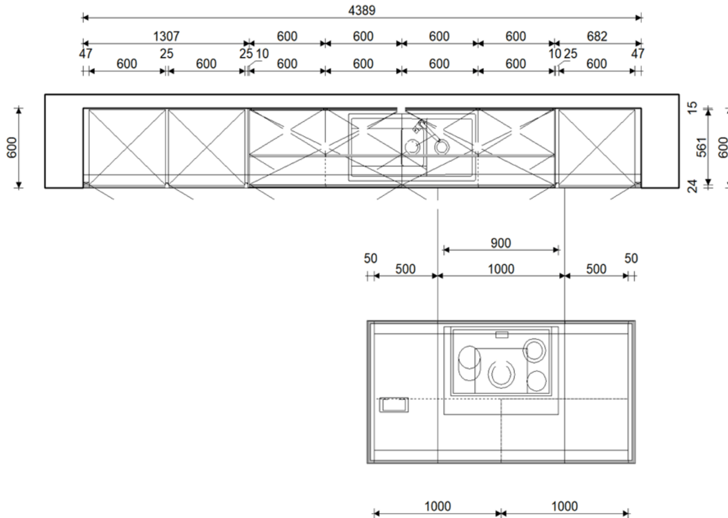
Musterküche RA-15
