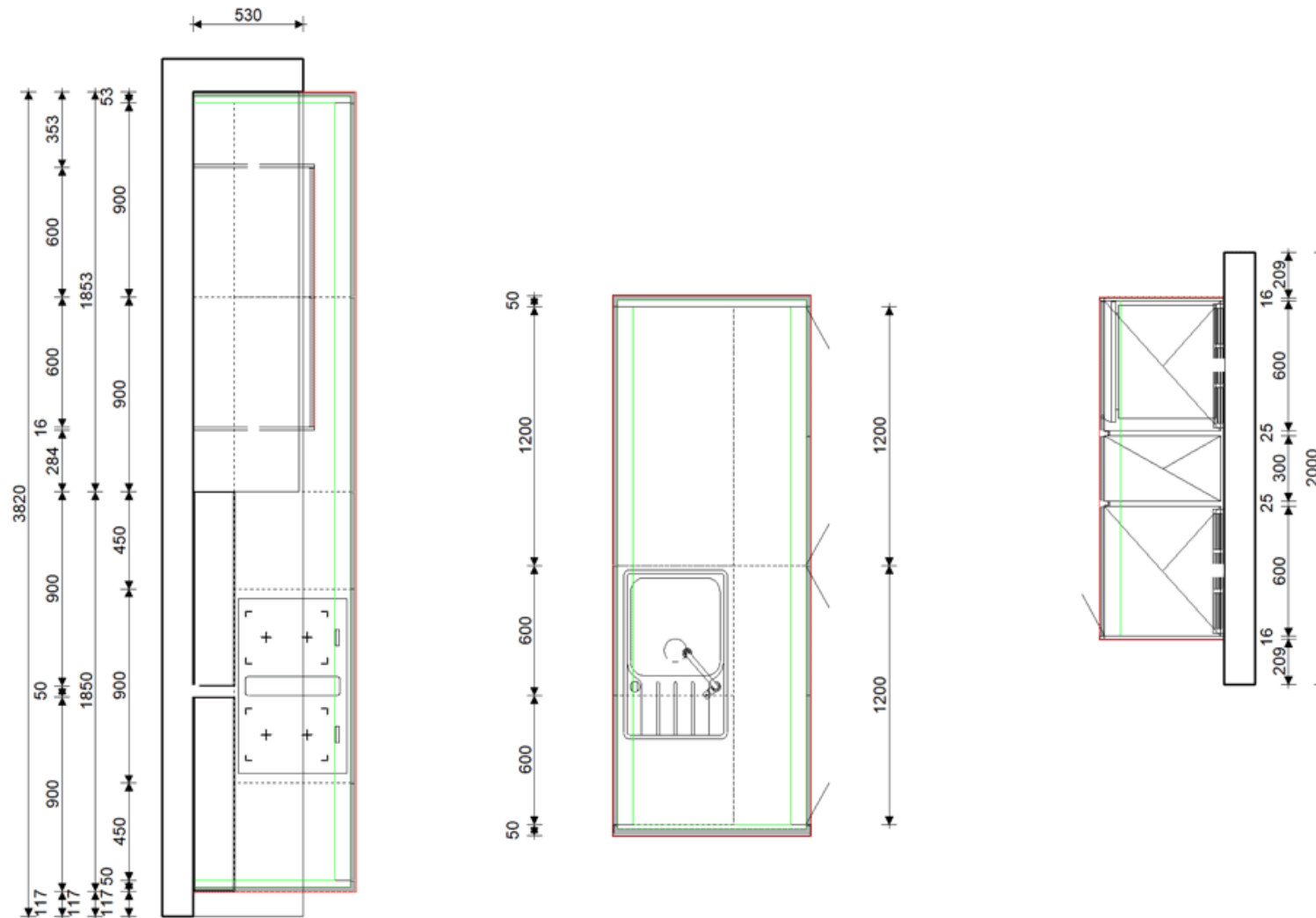
Musterküche OG-02
