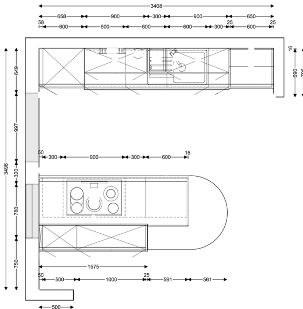
Musterküche OG-35
