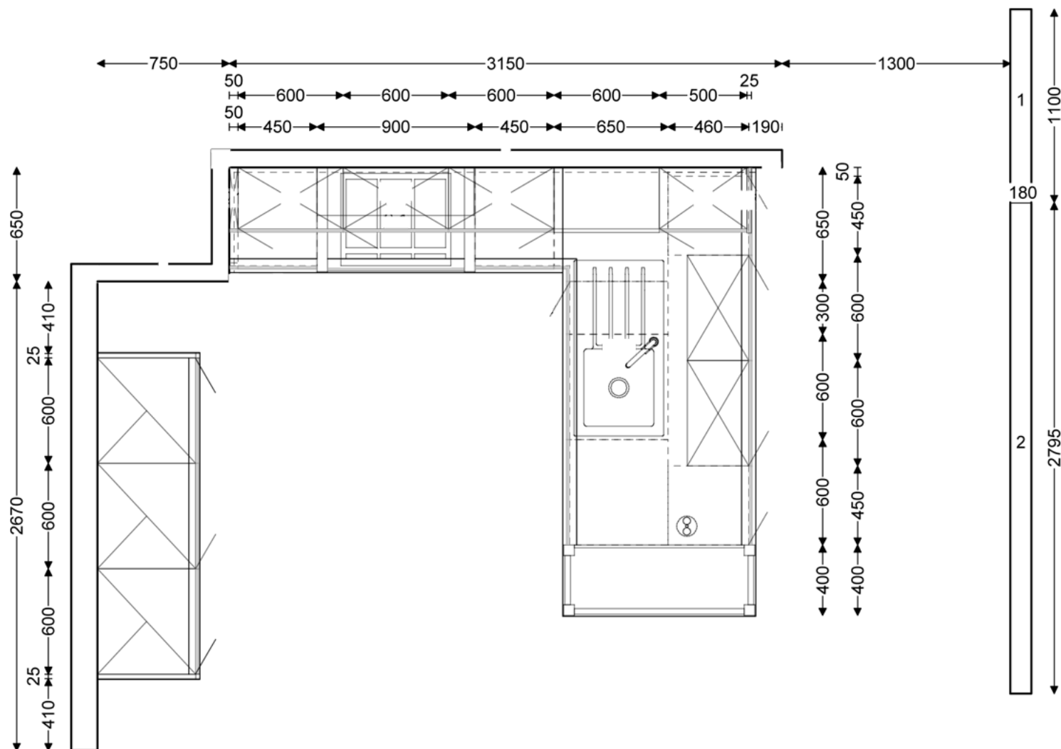
Musterküche KD-25
