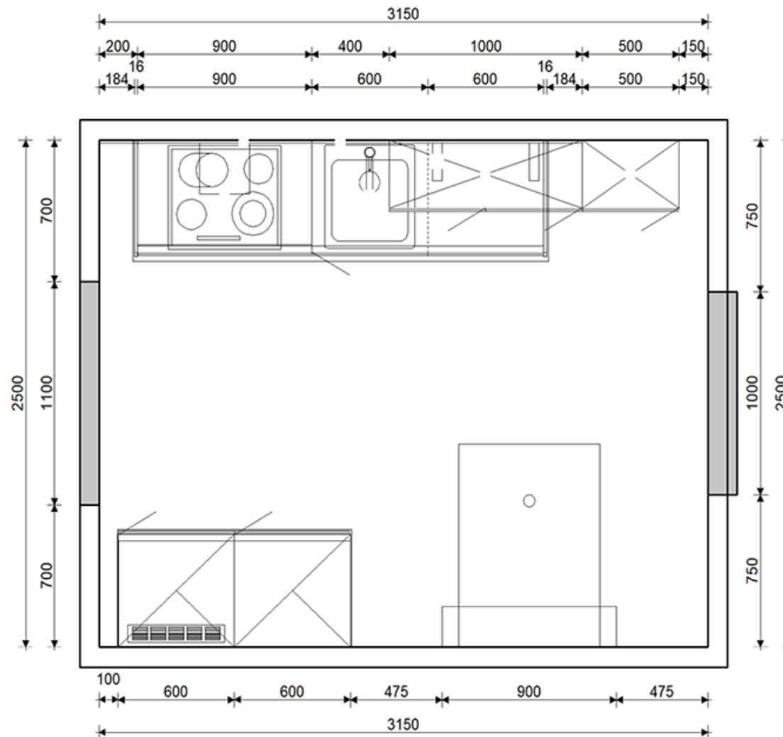
Musterküche KD-17
