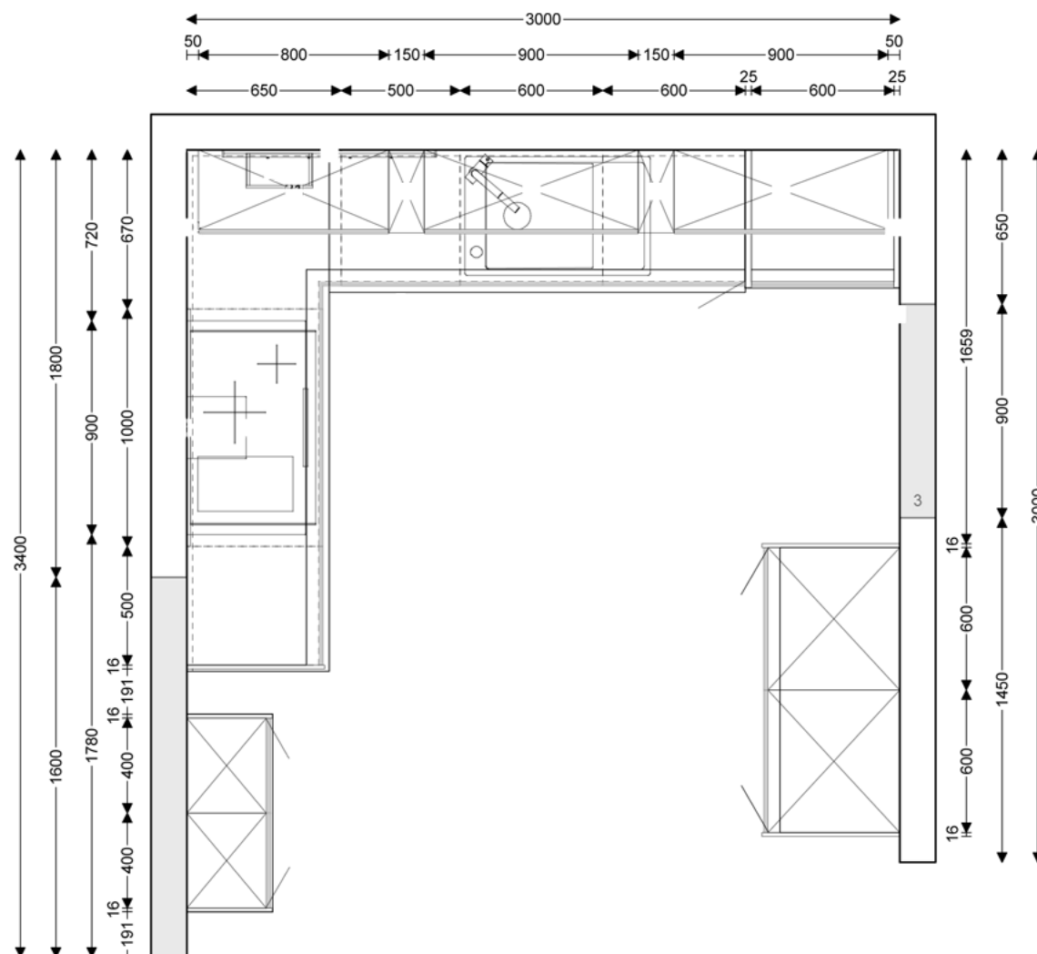
Cuisine d'exposition FR- MK-32
