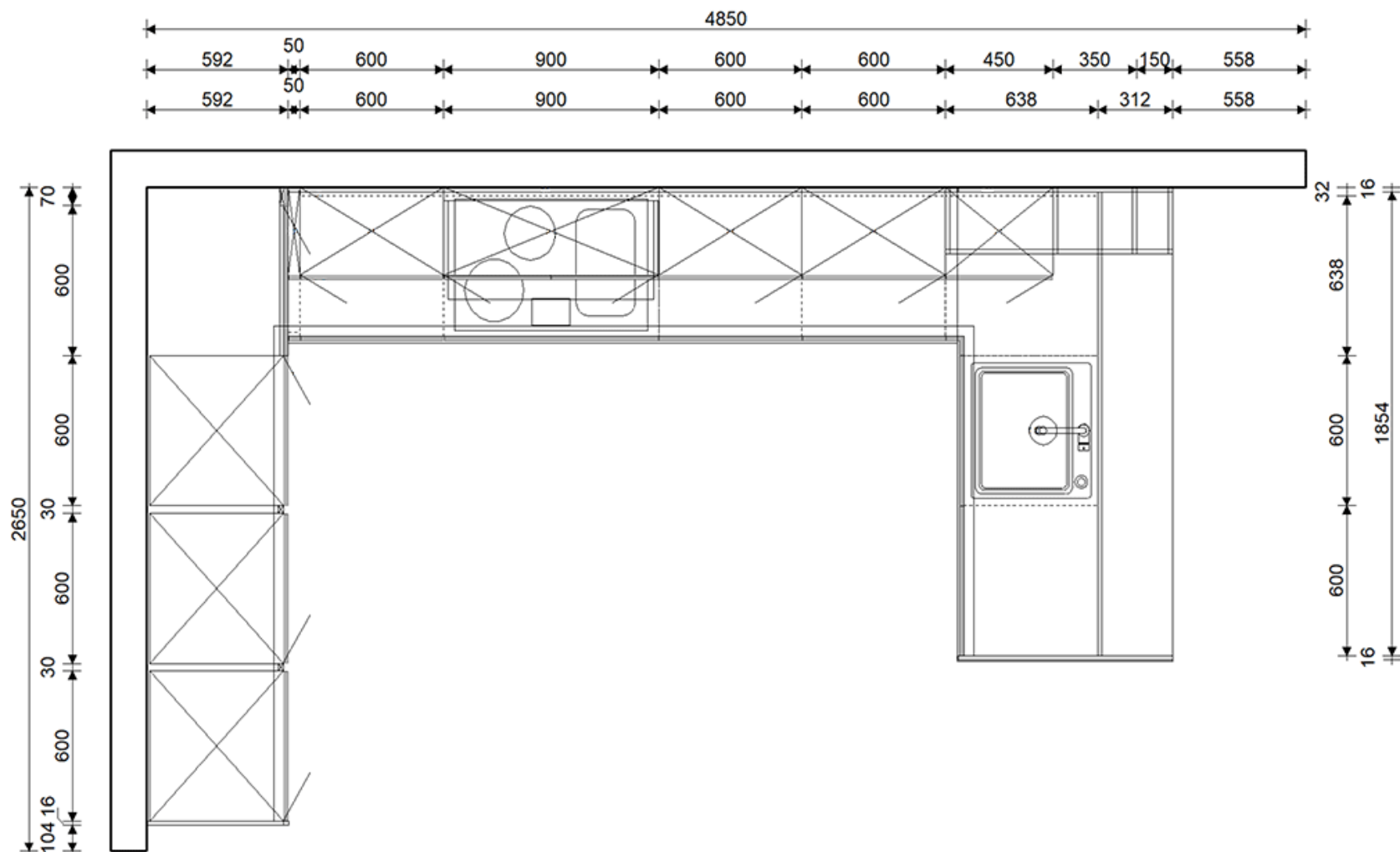
Cuisine d'exposition FR-MK-16
