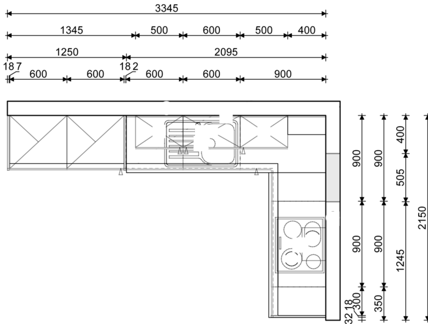
Musterküche BR-30
