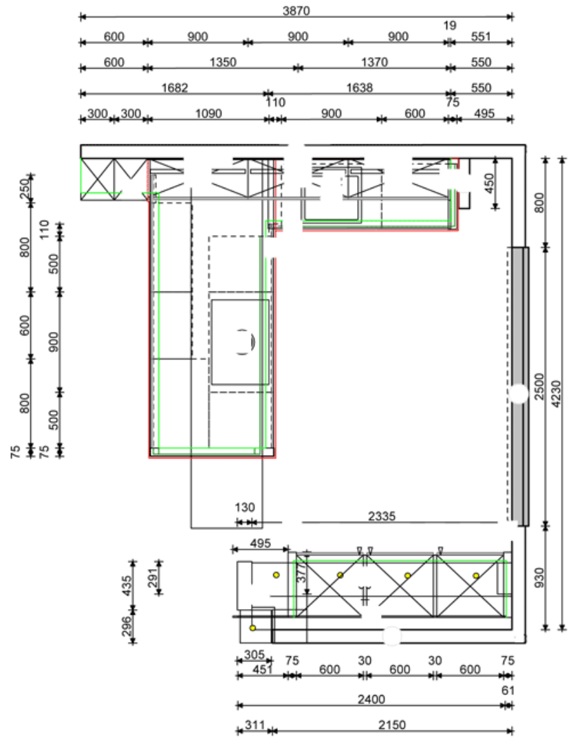
Musterküche BR-02
