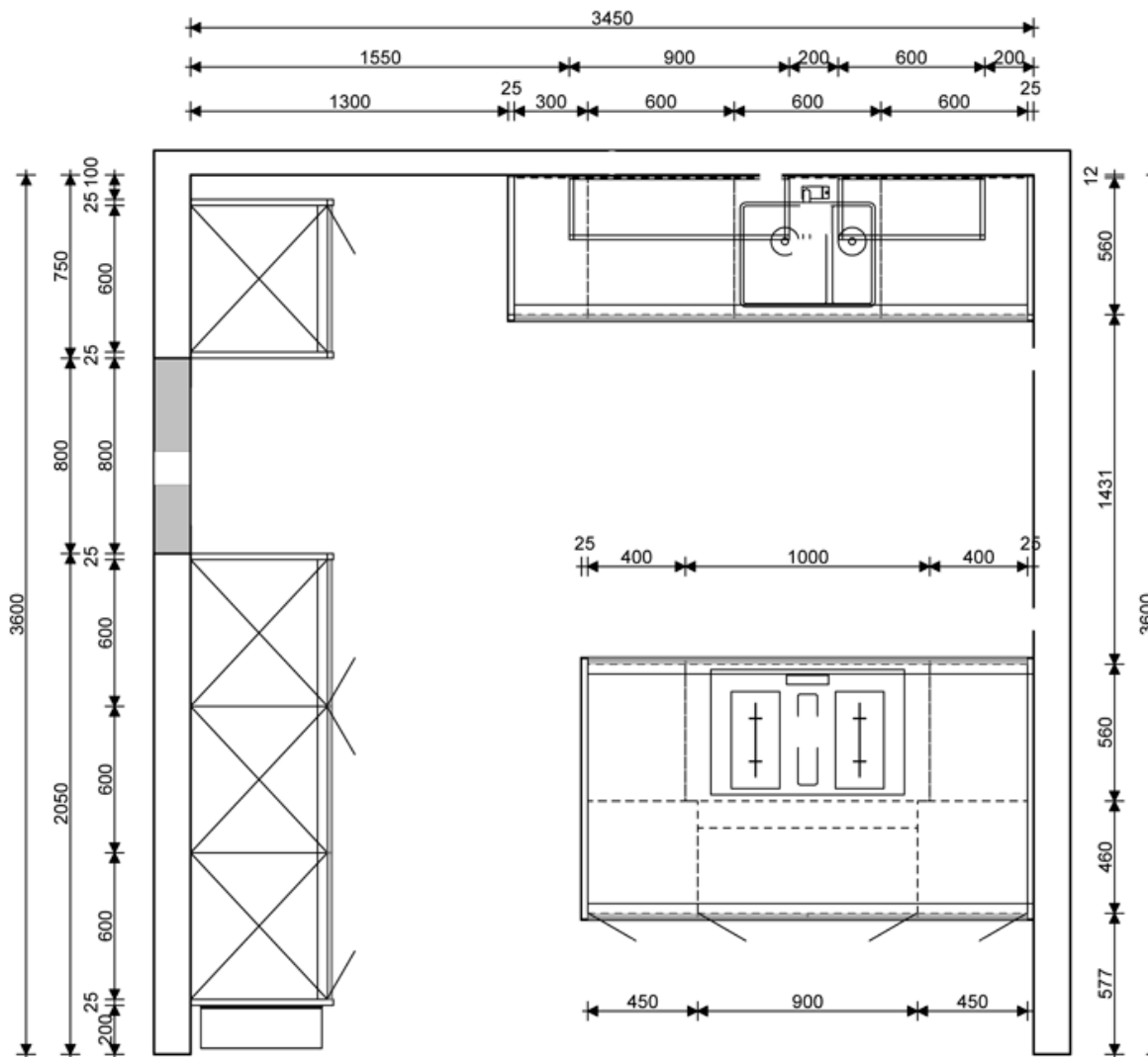
Musterküche BI-64
