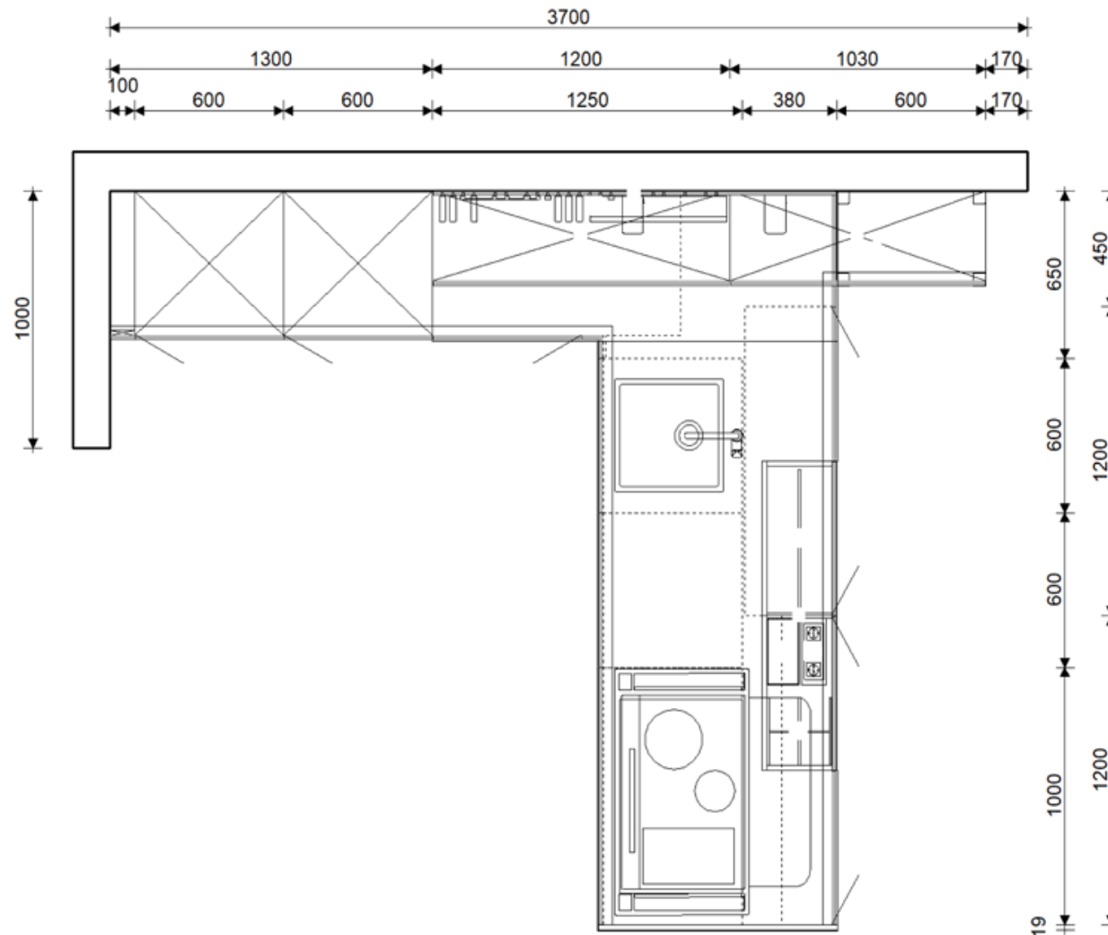
Musterküche BI-55A
