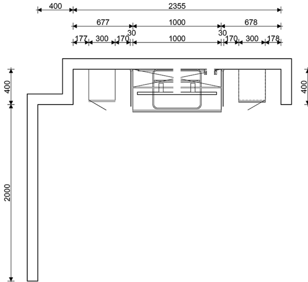
Musterküche BI-15B
