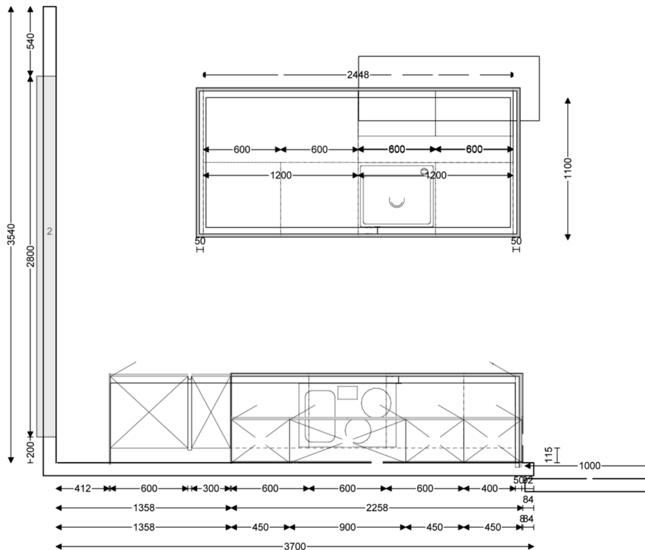
Musterküche BI-01
