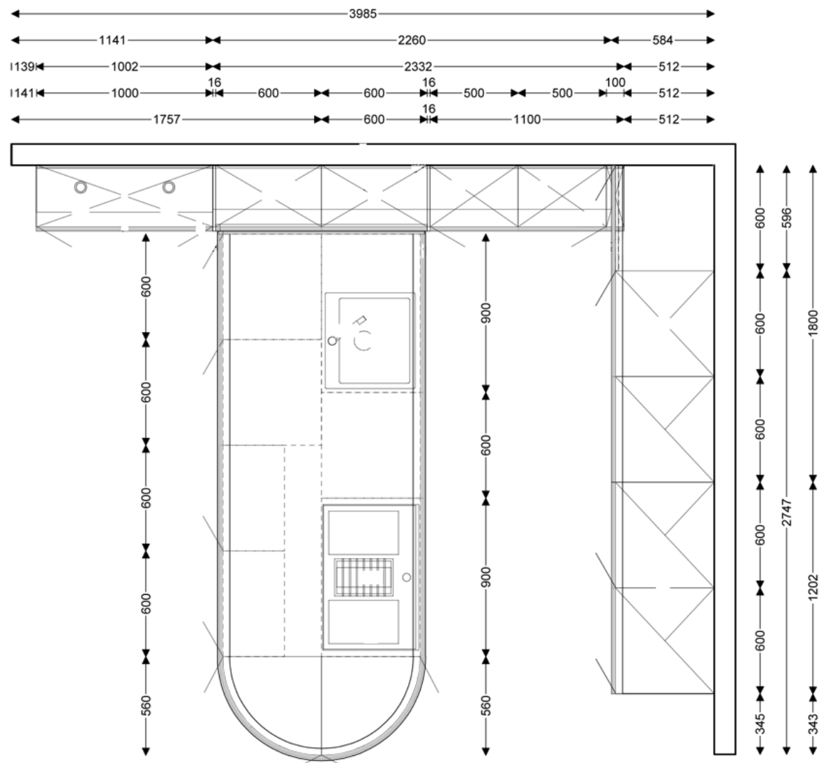
Musterküche BR-29
